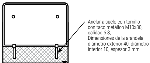
SECCIÓN D-D
