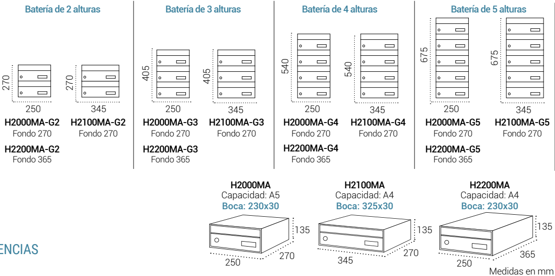
H2000MA (capacidad A5) H2200MA (capacidad A4)
