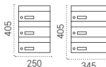
H4400AL-G3 Fondo 270 H4500AL-G3 Fondo 270 H4600AL-G3 Fondo 365
