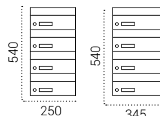
H4400AL-G4 Fondo 270 H4500AL-G4 Fondo 270 H4600AL-G4 Fondo 365
