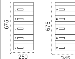
H4400AL-G5 Fondo 270 H4500AL-G5 Fondo 270 H4600AL-G5 Fondo 365
